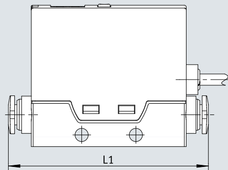
Dimensions – SFAE-...-Q4-...
